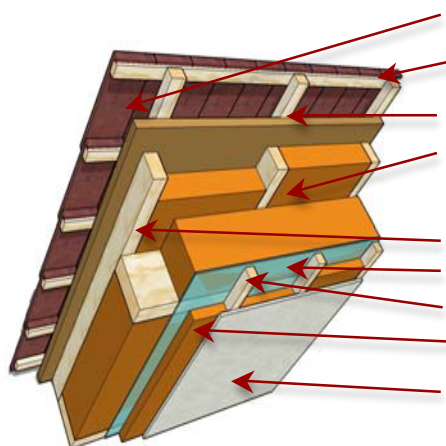
Toiture traditionnelle
