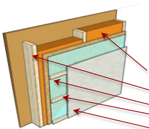
Mur maçonné
