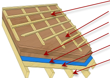
Toiture sarking
